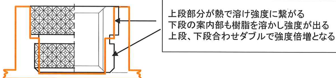
インサート熱圧入後状態
