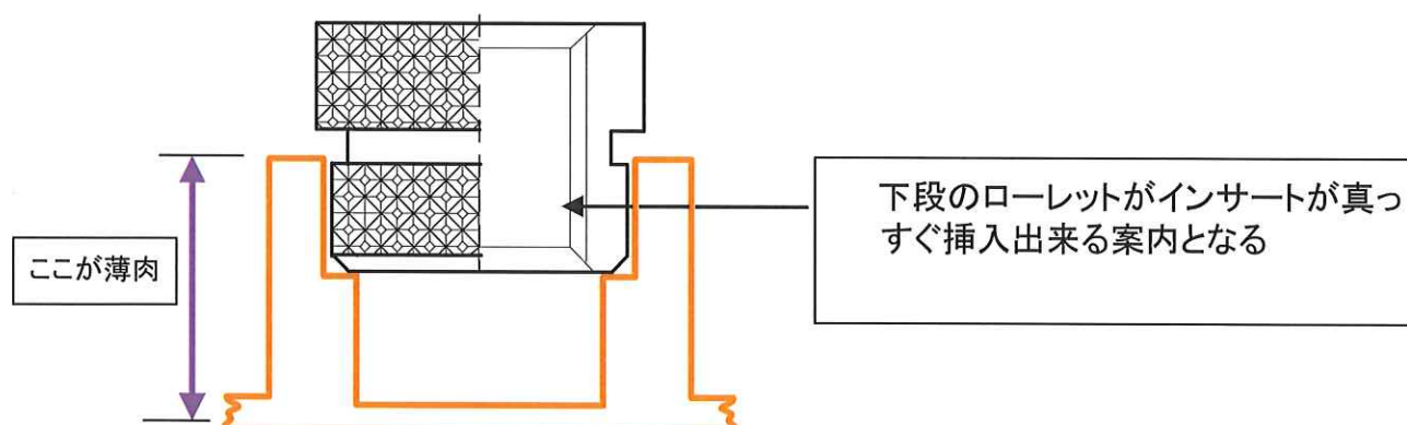
インサートがボス穴に仮置き状態
