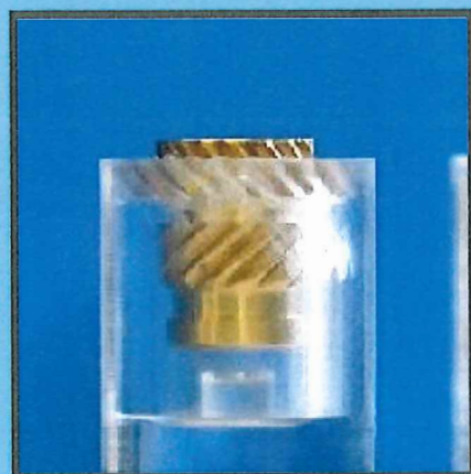
圧入後インサートの浮き沈み
