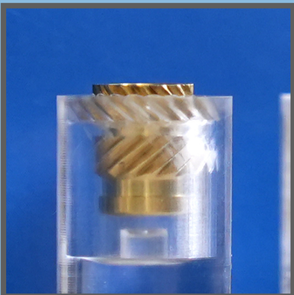
圧入後インサートの浮き沈み
