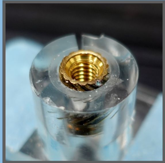
圧入後ボス割れ
